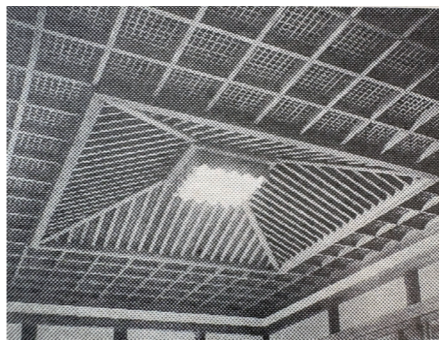
天窓に向かって四方から ついているものが上り竿ぶち (かんろだい物語より引用)
